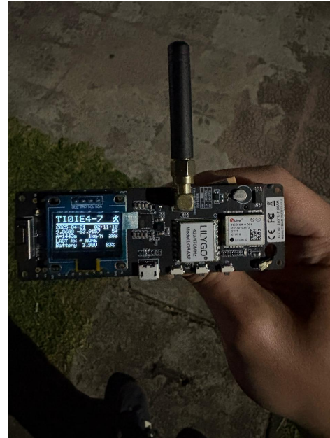
Figura 6: Tracker ESP32/LoRa operando
